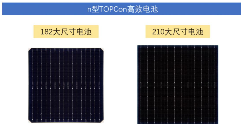
图 2：公司 n 型电池主要产品
